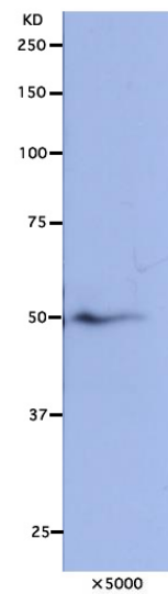
図 1. 細胞における Nuf2 タンパク質のウエスタンブロッティングによる検出 この抗体を 5,000 倍希釈して用いた。 ヒト Nuf2 タンパク質は 50kD のバンドとして検出された。
