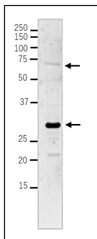
Fig. 2 抗-RPA (ヒト)抗体を使ったヒト 293 細胞抽出液中の内在性 RPA のイムノプロットによる検出
