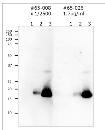
図2 抗 HIV-1 Gag p17 抗体 (65-008, 65-026) を用いたウェスタンブロッティングによる HIV-1 Gag p17 タンパク質の検出。
