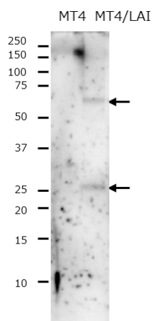
図2 抗 HIV-1 p24 抗体(65-023)を用いたウェスタンブロット法による p24 抗原の検出
